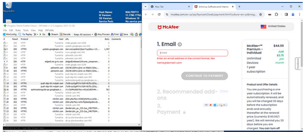
図 28：McAfee 紹介詐欺の Fiddler キャプチャ
